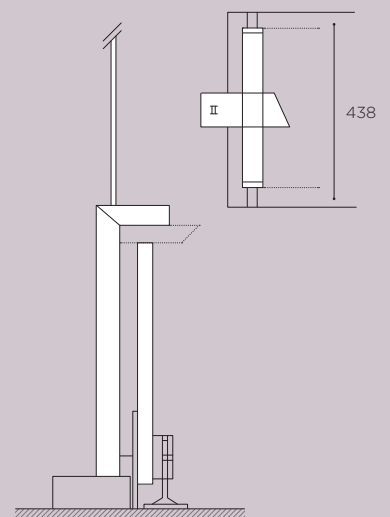
Assembly 5. Terminal. Conjunto 5. Remate frontal. Teilesatz 5: vorderes Abschlussstück.
