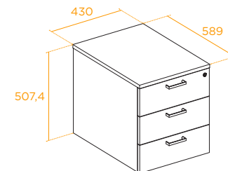
► Caisson hauteur bureau 3,3,3,3
