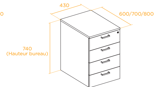
► Caisson hauteur bureau 3,3,3,3
