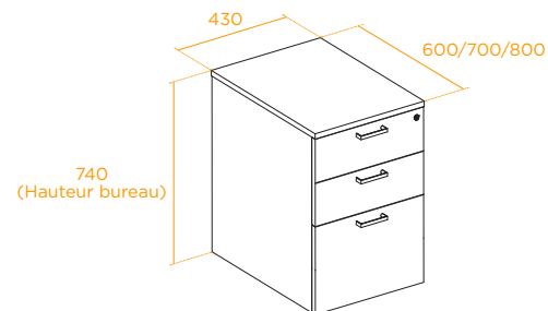
► Caisson hauteur bureau 3,3,6
